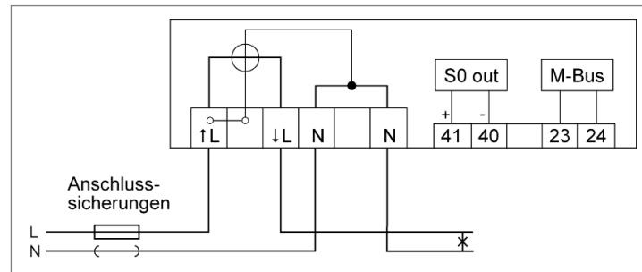
Bild 2: Vorsicherungen
